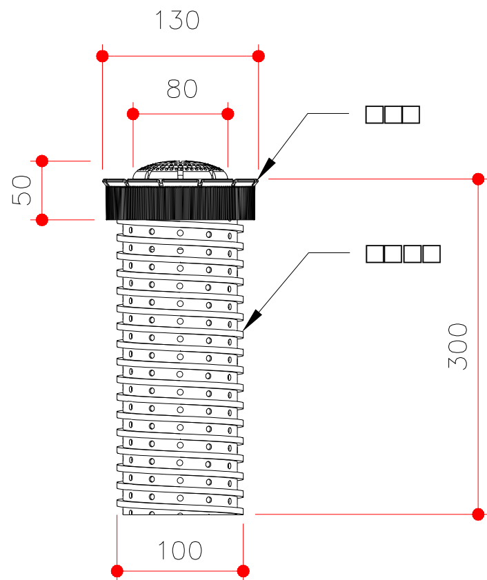
4 생육삼통관 정면도 SCALE = NONE
