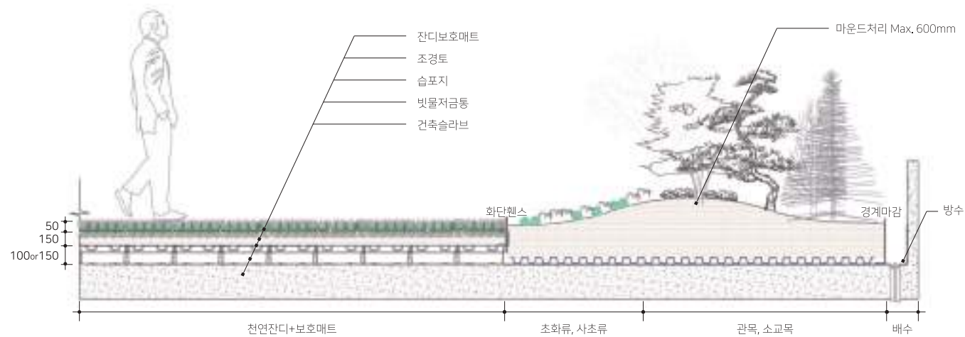
시공 단면도
