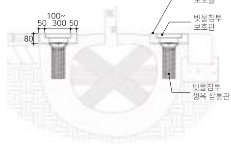
시공 단면도
