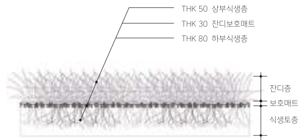
시공 단면도
