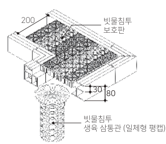
부분 상세도
