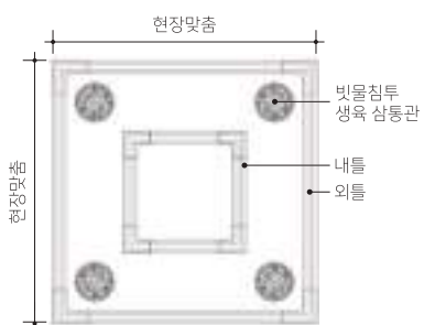
내부 평면도
