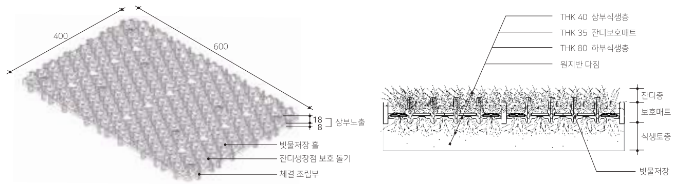
상세도
