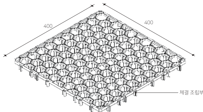
상세도
