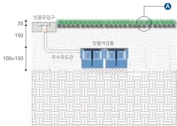
시공 단면도
